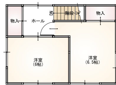
2階 平面図 S:1/100
