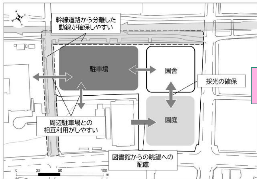
■建物配置図■
