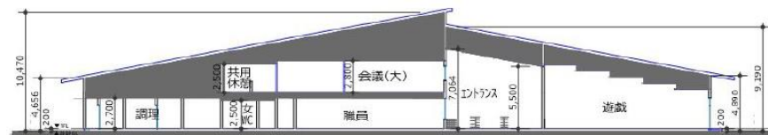
A-A断面図
